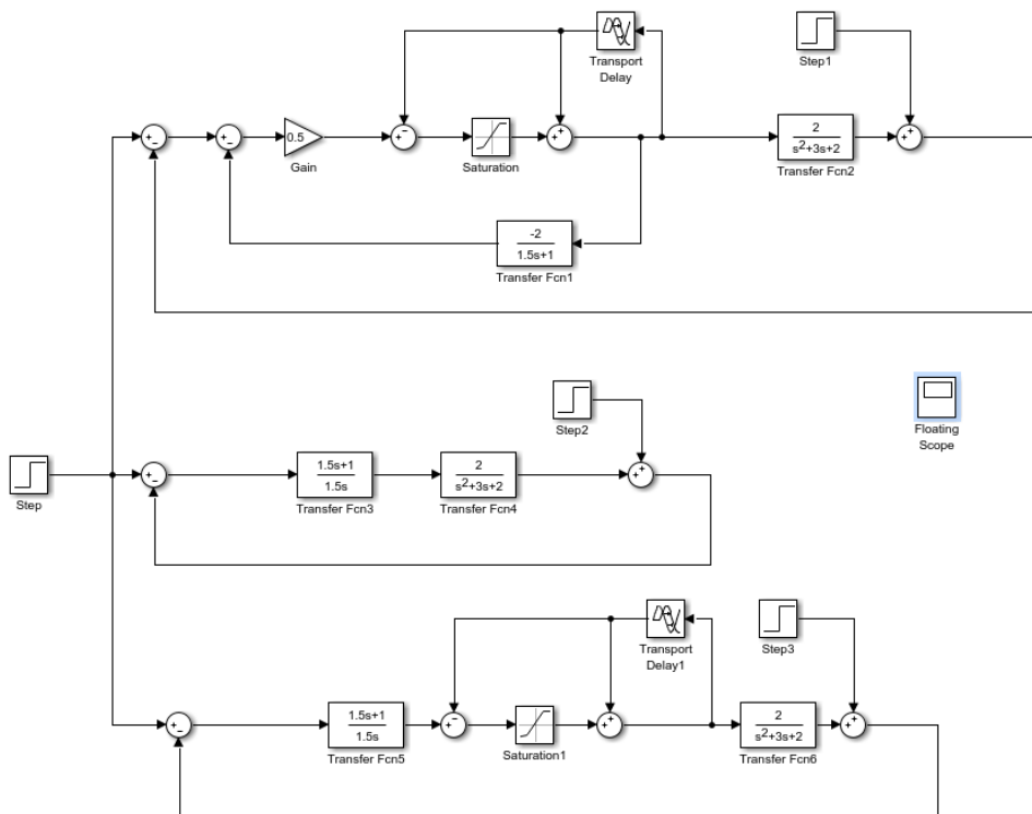
例 3 Simulink
