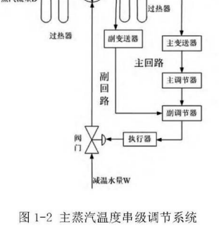
图 1-2 主蒸汽温度串级调节系统
