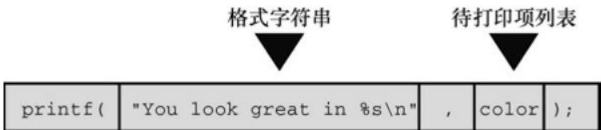
图4.6 printf()的参数
