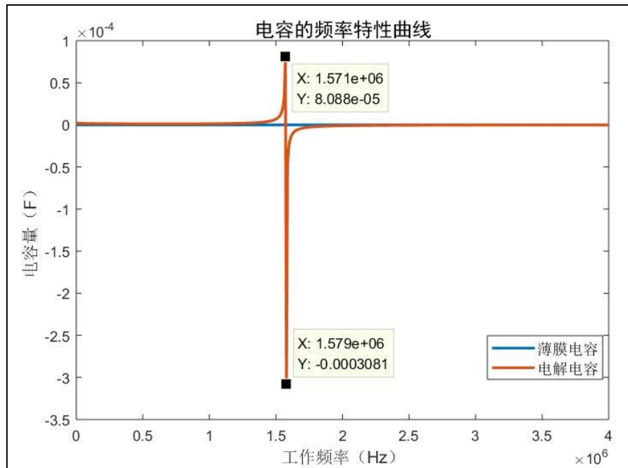
图 1-16 电容频率特性曲线示例图
