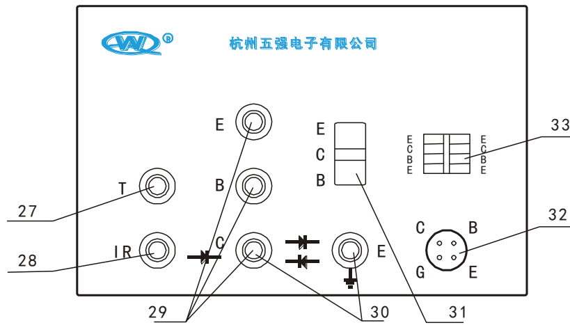
测试台面板示意图
