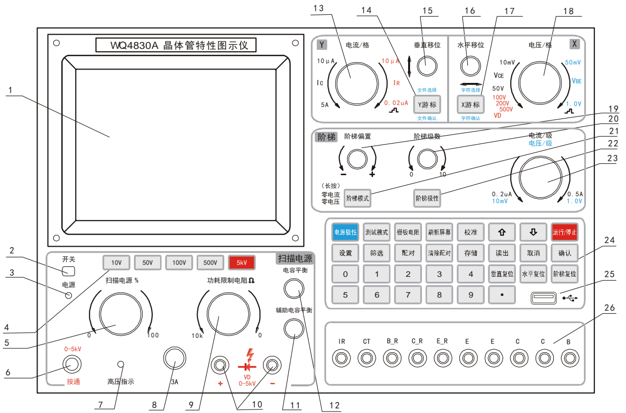
主面板示意图
