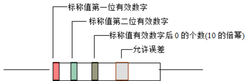
图 1-1 四色环电阻器示意图
