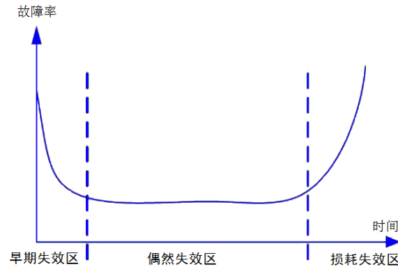
图 1- 11 电子元器件的效能曲线
